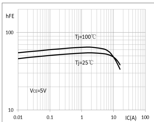
hFE - I_C (BA16N25A)
